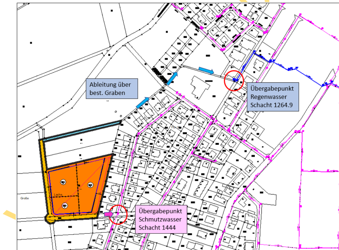
Abbildung 5: Entwässerung
